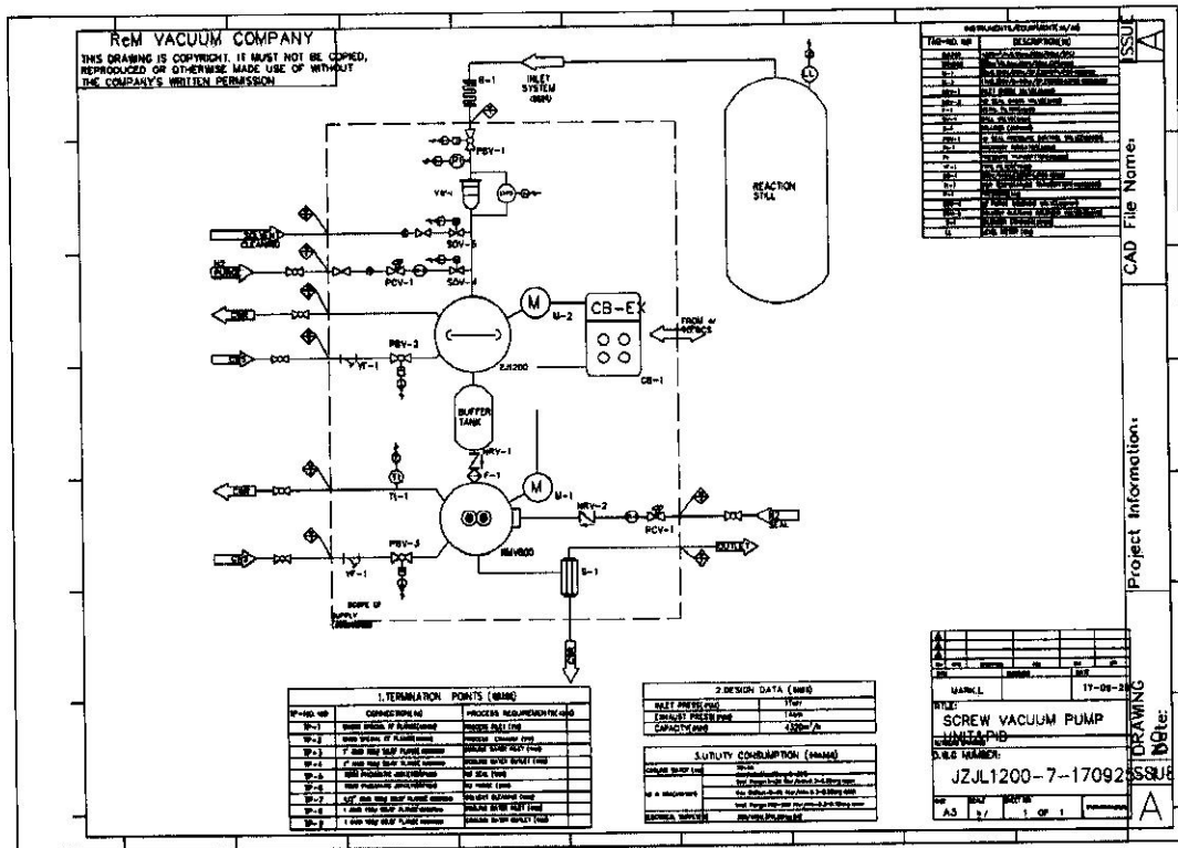
总装图（仅供参考）
